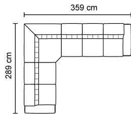
067 SECT. 00+01+11+01+01+02
